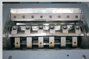
RG-56E 片刀型 Paddle blades type
