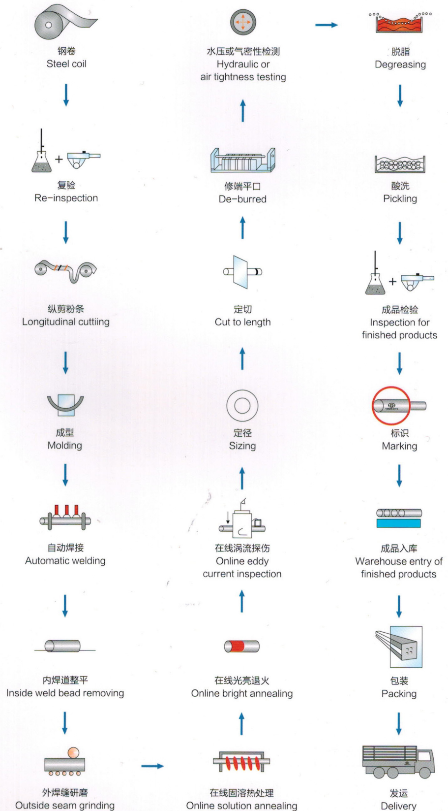
连续成型生产工艺流程图 (生产线设备产品)
