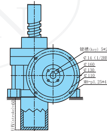
T型 (顶板式) T type (top plate)
