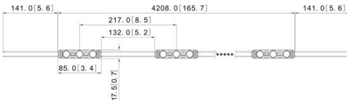
单位: mm(in)
