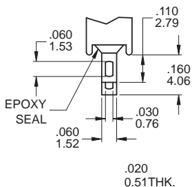
M1 Solder lug
