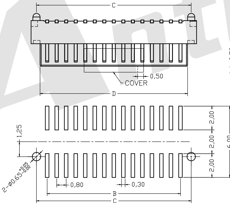
P.C.B PATTEN
