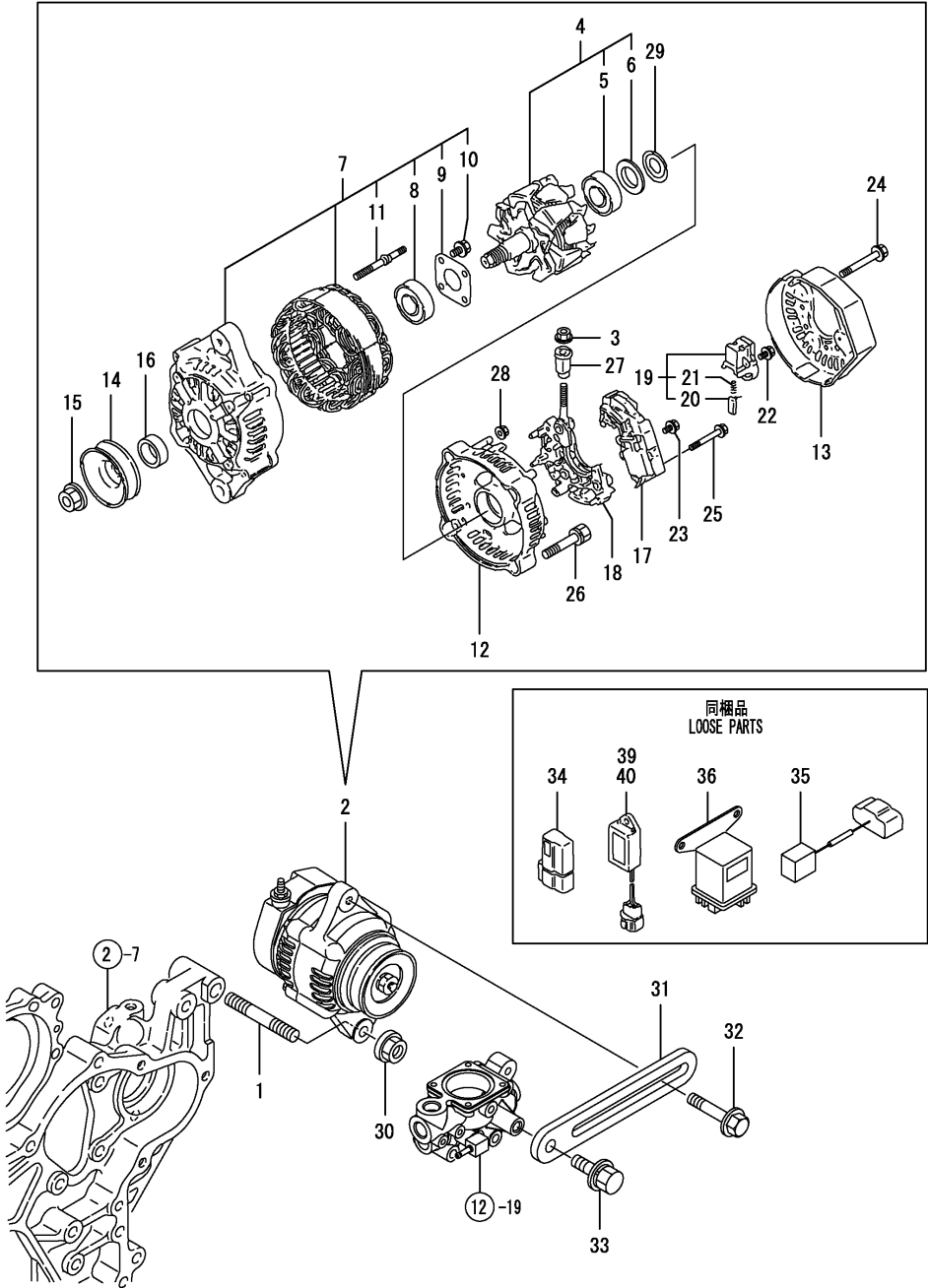
Fig.18. GENERATOR
